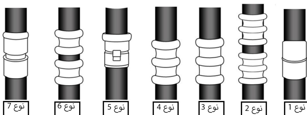
تصویر ۷- انواع اتصالات ستون‌های چادر به یکدیگر در نگاره‌ها. منبع: (نگارندگان)
