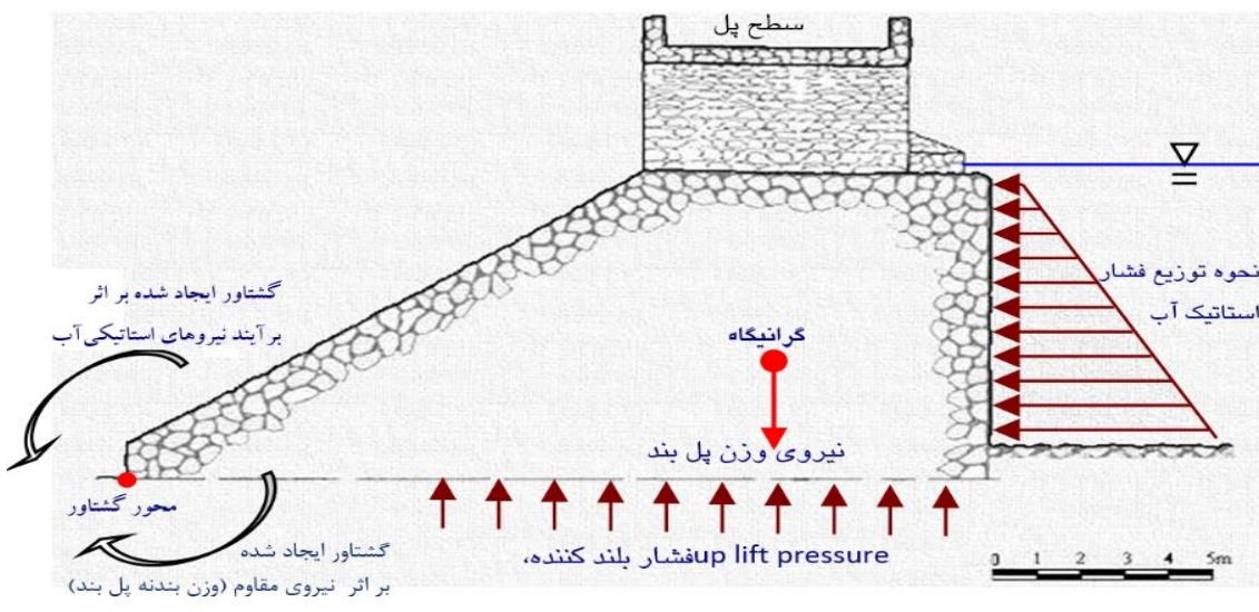
تصویر ۱۳- برش عرضی پل بند امیر؛ نیروهای وارد بر پل بند. منبع: (نگارنده)
